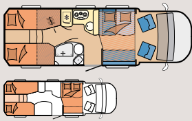
T75 HGE
