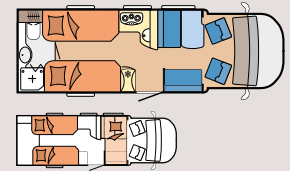
T70 E
