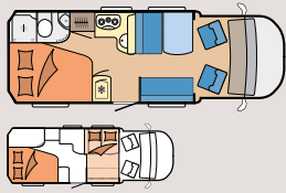
T65 FL
