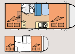
A60 GF
