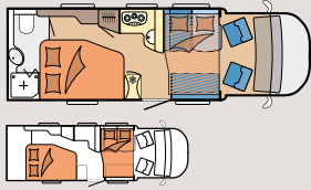
T75 HF
