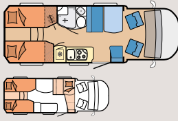
T65 GE
