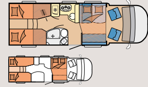
T75 HGE
