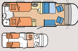
T70 E
