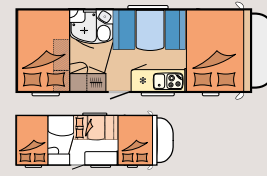
A70 GM
