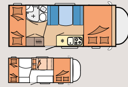
A65 GM
