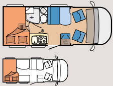
V60 GF
