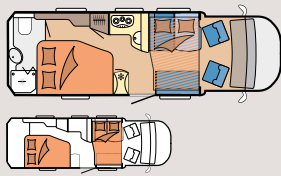
T75 HF
