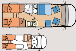
V65 GE
