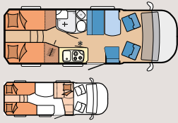
V65 GE
