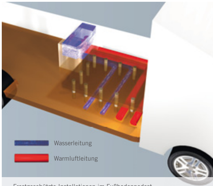
Frostgeschützte Installationen im Fußbodenpodest
